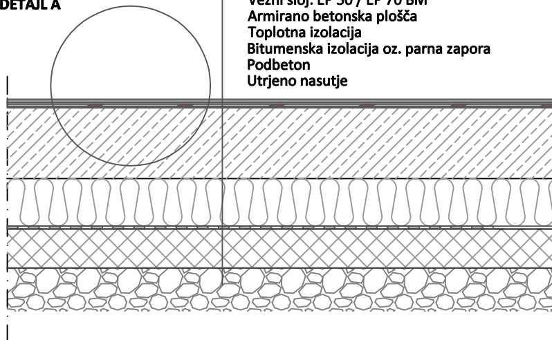
DETAJL A
