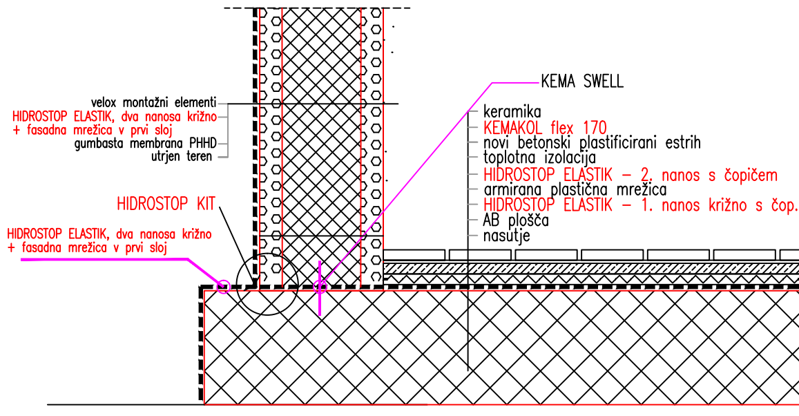
DETAJL A
