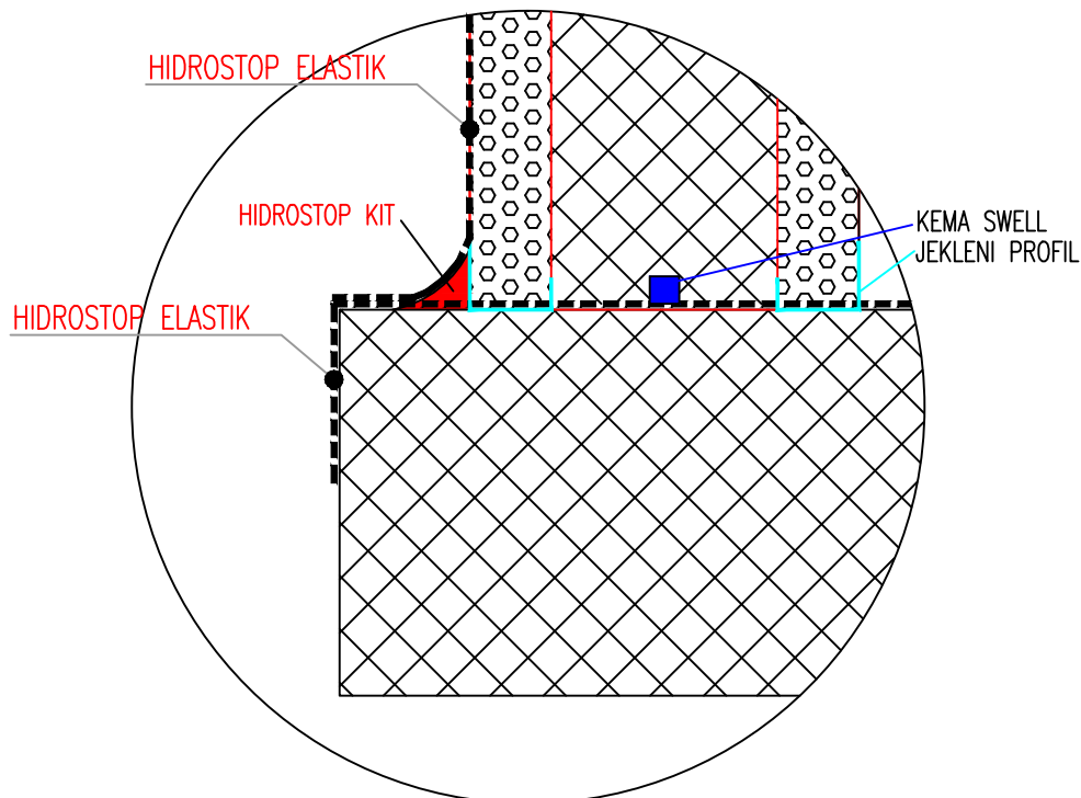
DETAJL A
