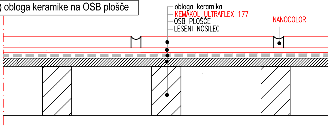
D) obloga keramike na impregnirano iverko
