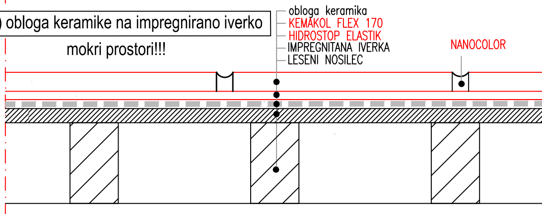
C) obloga keramike na OSB plošče
