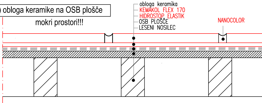
B) obloga keramike na impregnirano iverko
