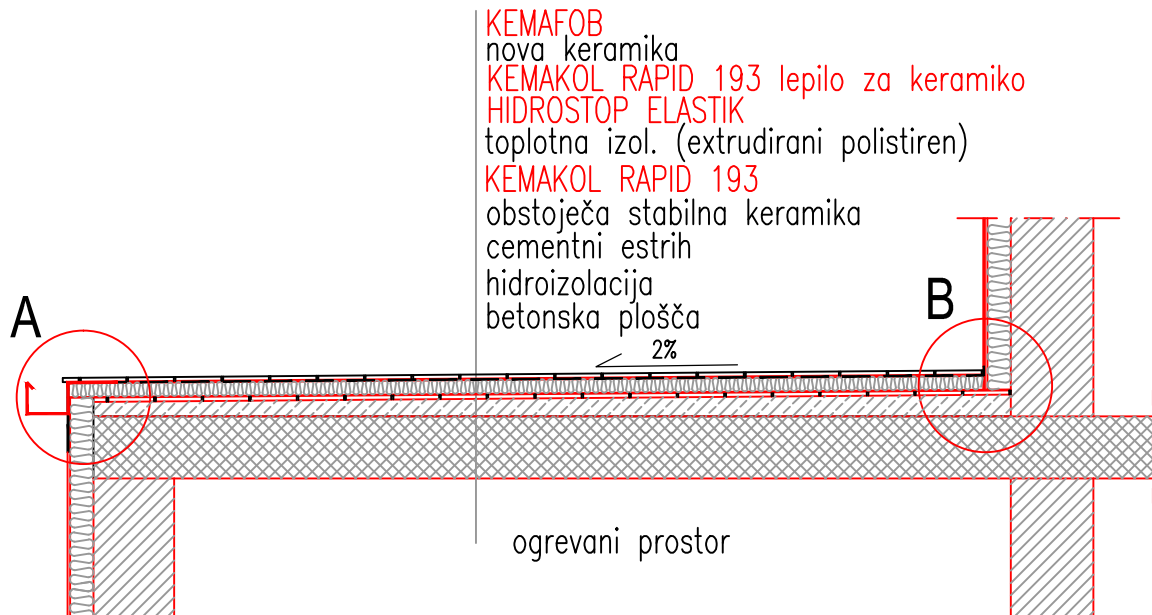
DETAJL A
